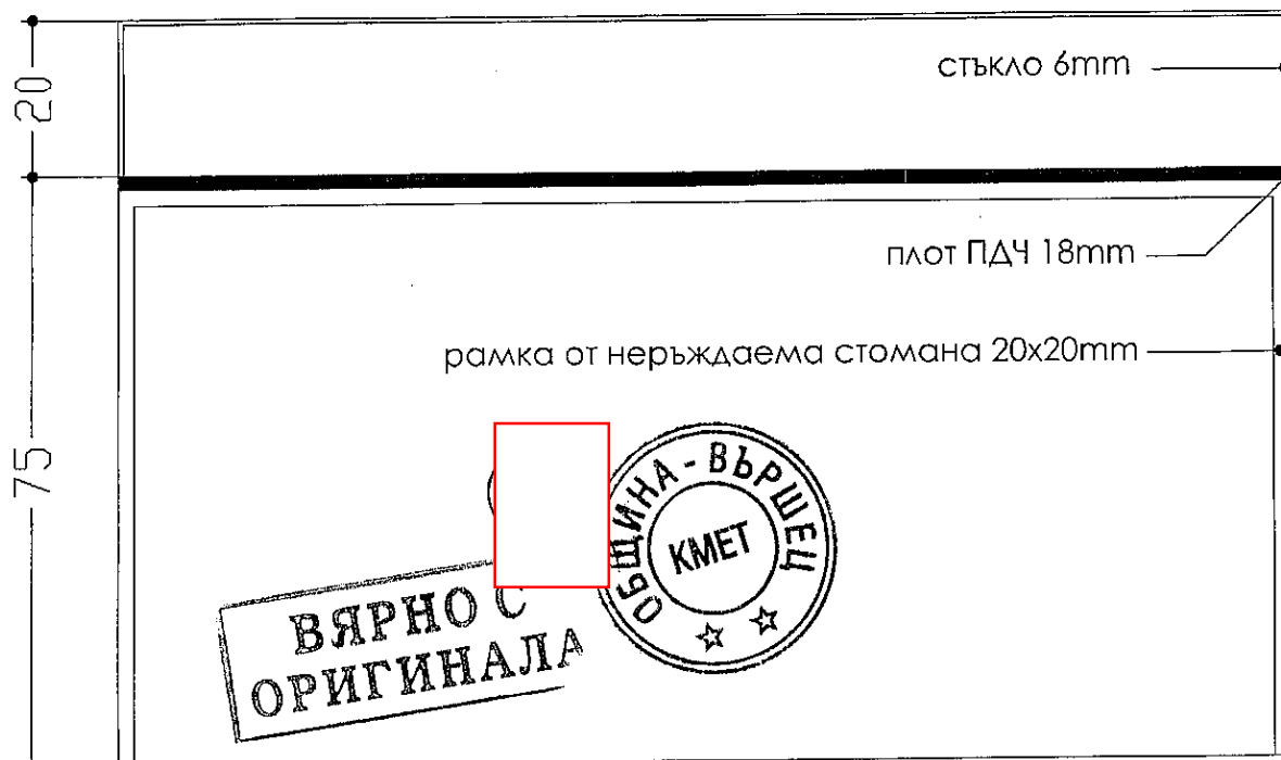
ИЗГЛЕД
